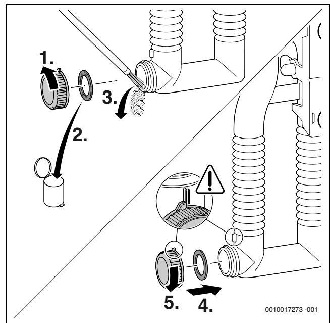
Fig. 53 Pulizia del sifone per la condensa
