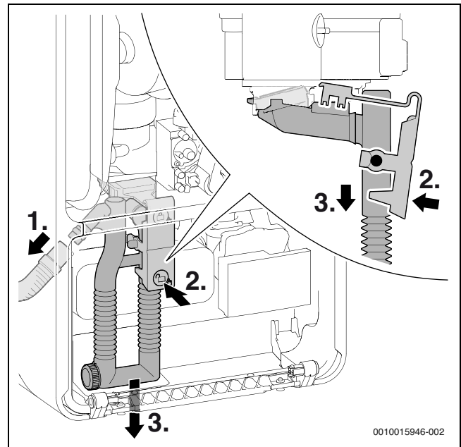
Fig. 52 Smontaggio del sifone per la condensa
