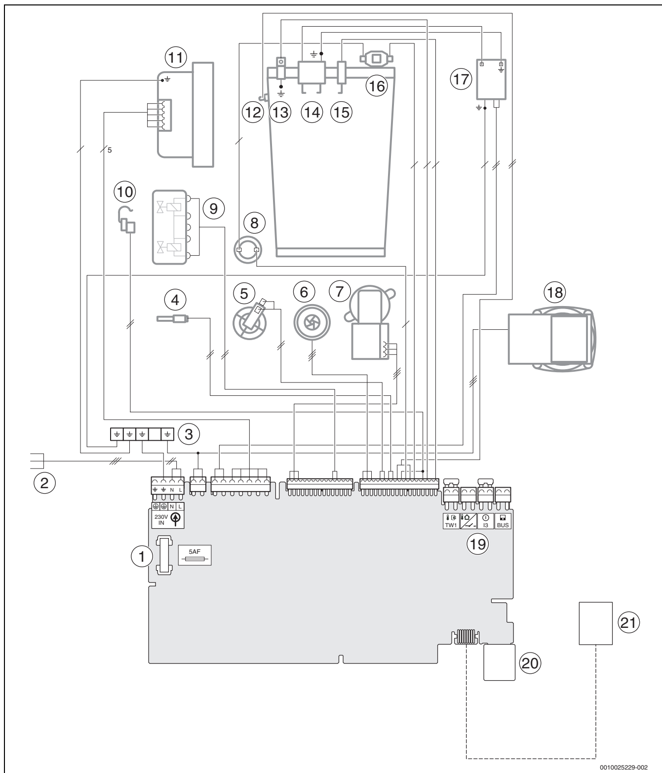
Fig. 73 Cablaggio elettrico
