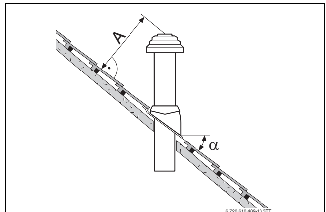
Fig. 6 Distanze ed inclinazione con tetto inclinato
